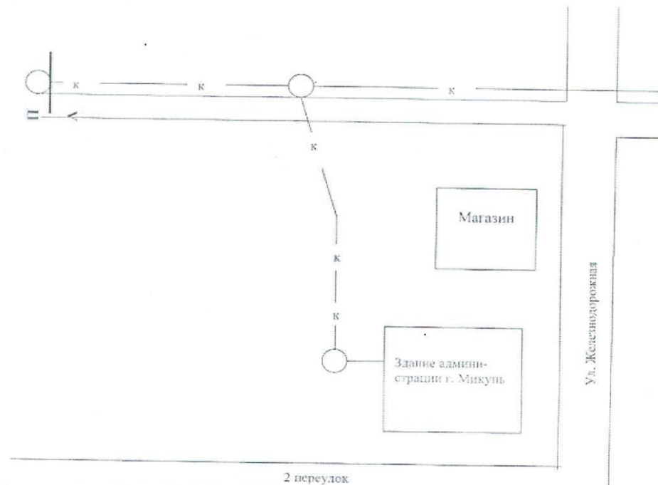
Схема сетей водоотведения администрация ГП «Микунь».
