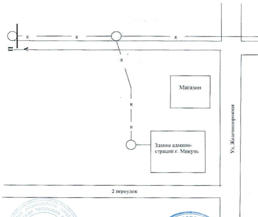
Схема сетей водоотведения администрация ГП «Микунь».
